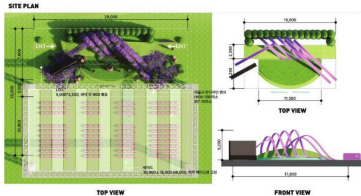
메인무대 평면도 및 상세도
